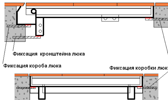
Схема монтажа люка и укладки плитки на люк
